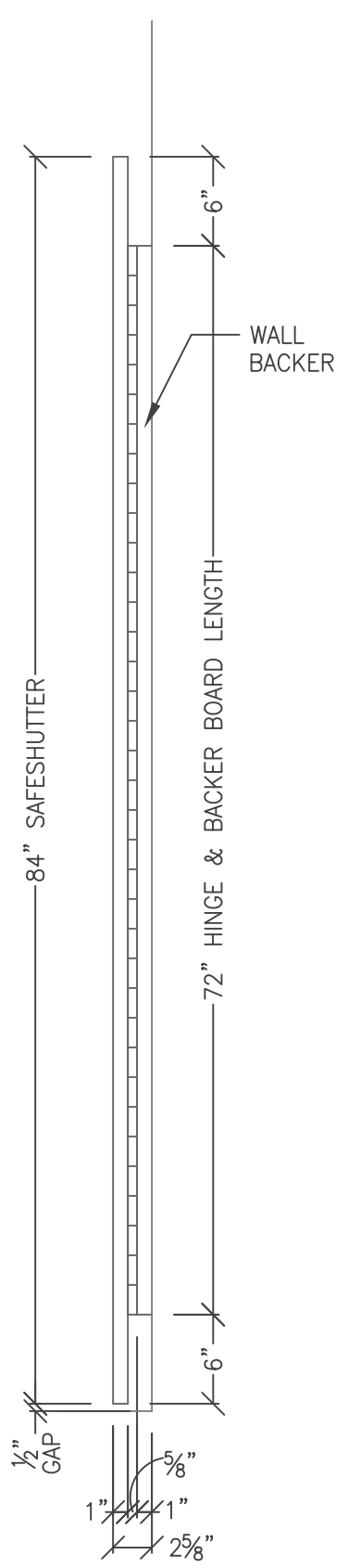
2 ELEVATION 2.7 SCALE: 1" = 1'-0"
