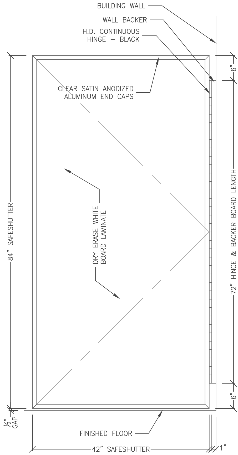
1 ELEVATION 2.7 SCALE: 1" = 1'-0"
