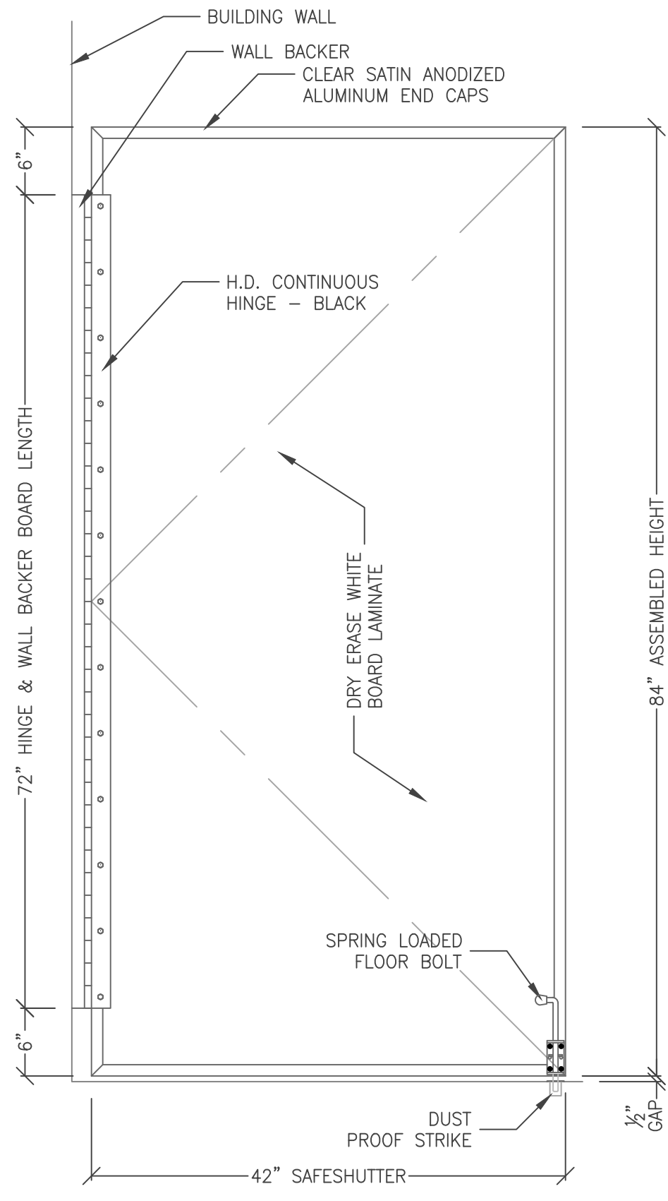
3 ELEVATION 2.7 SCALE: 1" = 1'-0"
